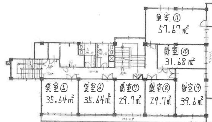
(3階)
